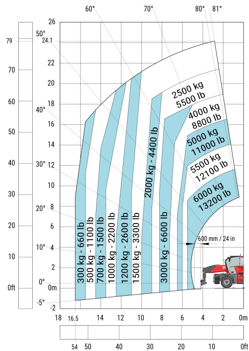
Stroj na pneumatikách s vidlicou
