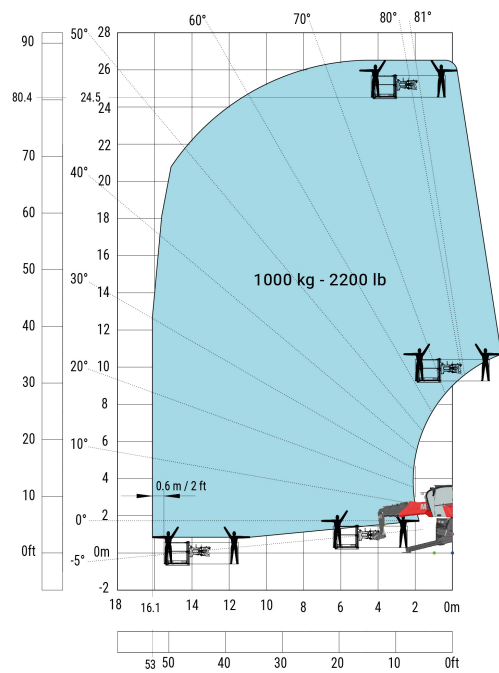
Otáčanie s vysokozdvížnou plošinou s hmotnosťou 1 000 kg na spustených stabilizátoroch
