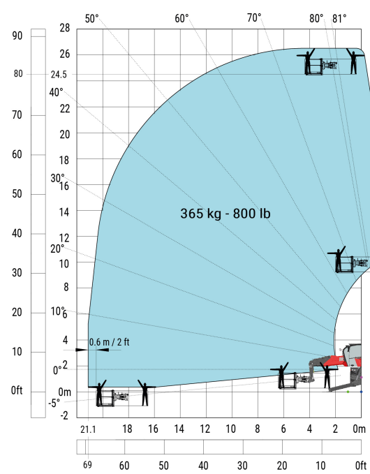
Otáčanie s vysokozdvížnou plošinou s hmotnosťou 365 kg na spustených stabilizátoroch
