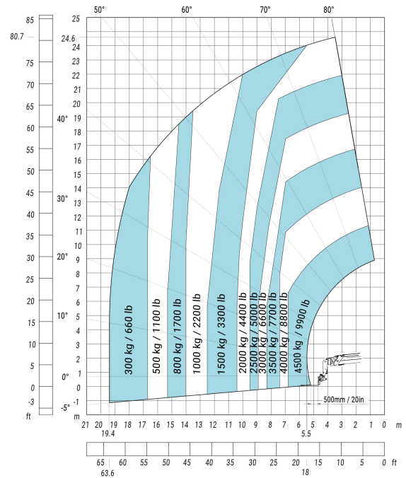
Otáčanie s vidlami na spustených stabilizátoroch
