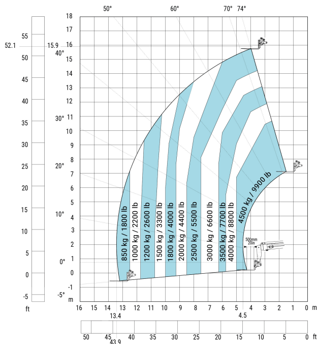
Otáčanie s vidlami na spustených stabilizátoroch
